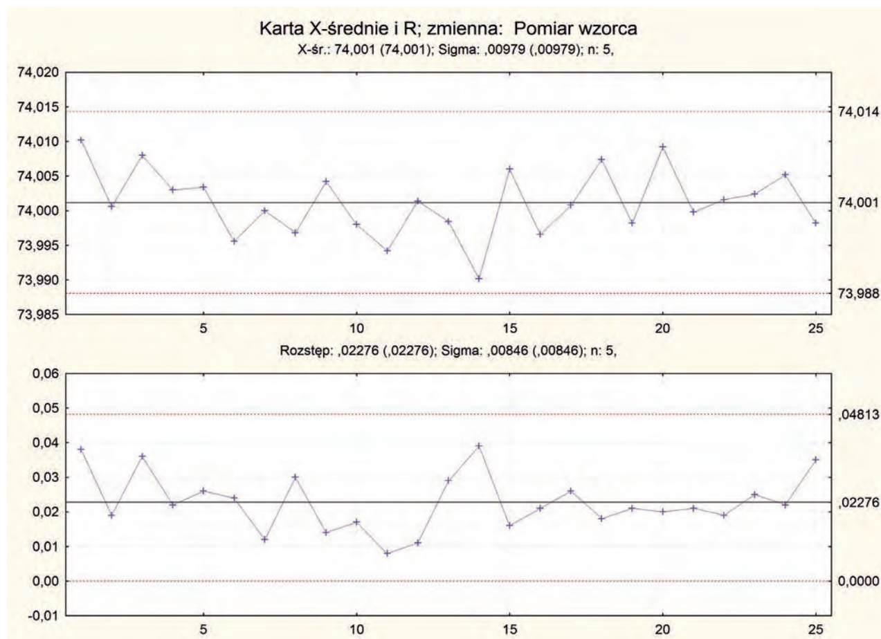
Rys. 8. Karta kontrolna otrzymana w STATISTICA
